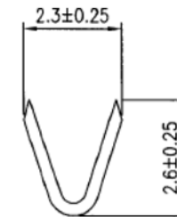
A-A SECTION
